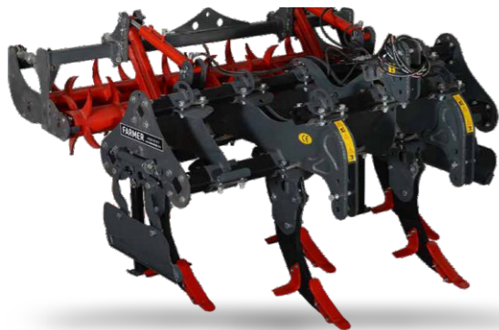
Cizel Partlatma ağır italyan
